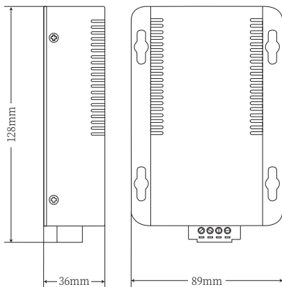
图2 产品尺寸图
