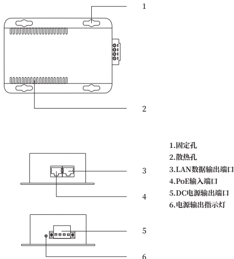
图1 产品示意图
